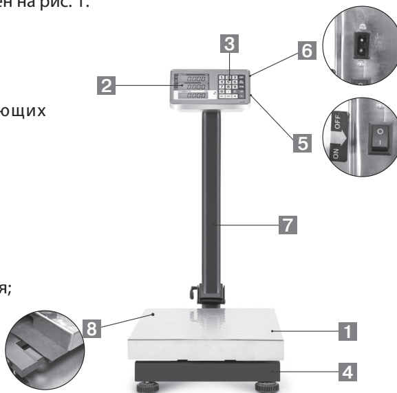
Рис. 1. Весы торговые электронные «М-ER 335AC(L)P(U)»
