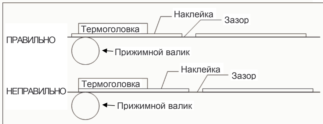
Рисунок 1.20 – Варианты правильной и неправильной положения ленты этикеток
