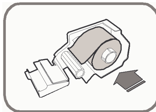
Рисунок 1.15 – Установка нового рулона
