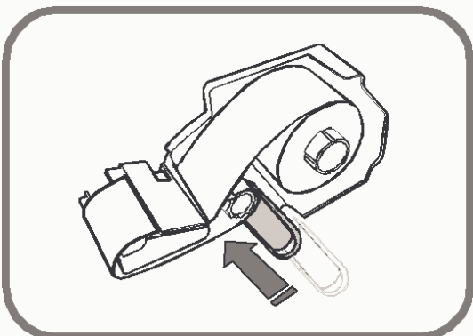
Рисунок 1.17 – Фиксация ленты на приёмной катушке
