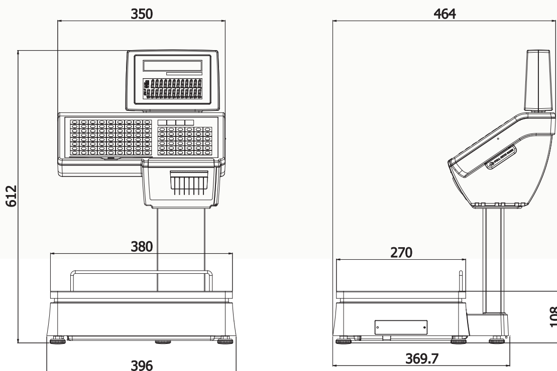
Рисунок 1.1 – Вид весов CL5000-D в геометрической проекции
