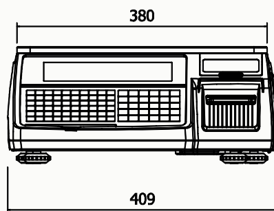
Рисунок 1.2 – Вид весов CL3000-B в геометрической проекции
