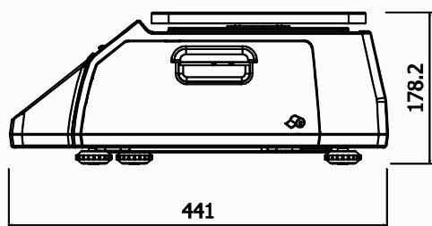
Рисунок 1.2 – Вид весов CL3000-B в геометрической проекции
