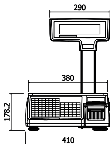
Рисунок 1.3 – Вид весов CL3000-P в геометрической проекции
