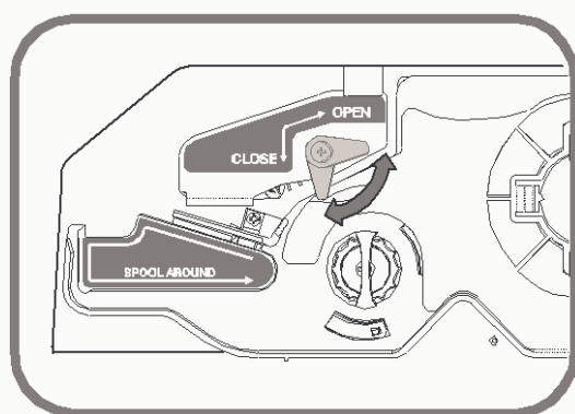
Рисунок 1.21 – Натяжение ленты
