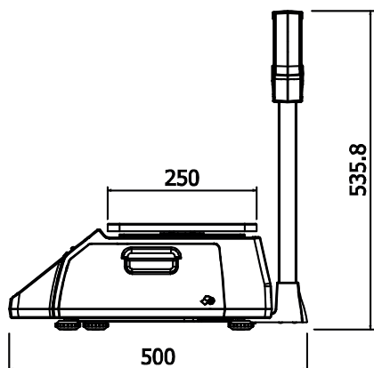
Рисунок 1.3 – Вид весов CL3000-P в геометрической проекции
